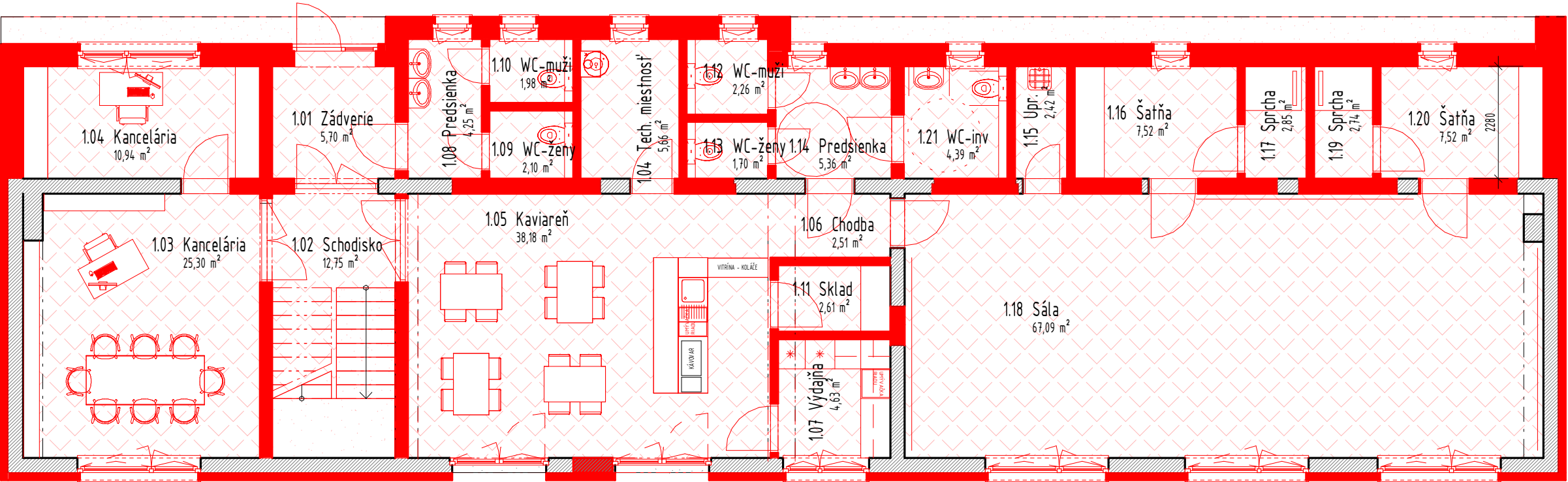
Pôdorys 1 NP
